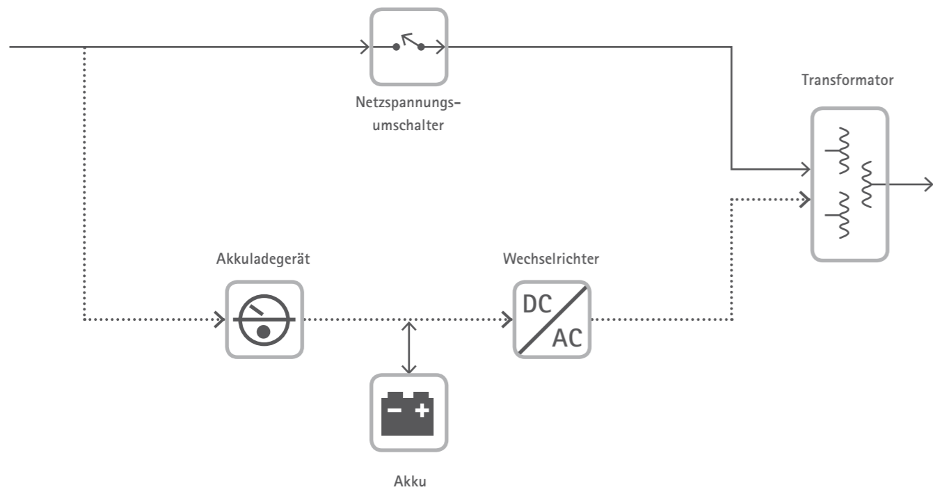
Abb. 5.2: Netzinteraktive-USV (Klasse 2)
