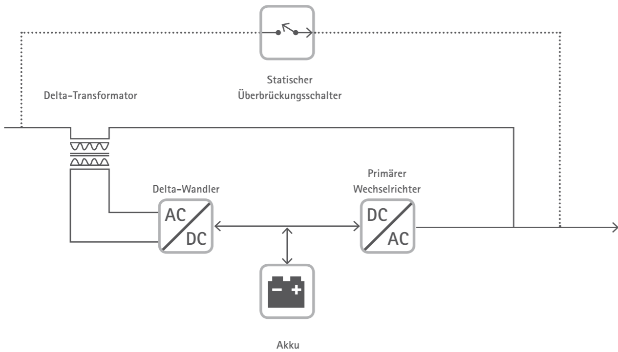
Abb. 5.3: Online-USV (Klasse 1)
